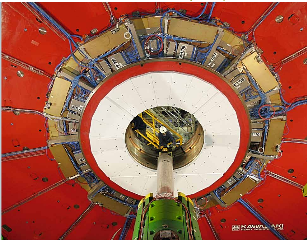
Montáž CMS detektoru, součásti obřího urychlovače částic CERN
